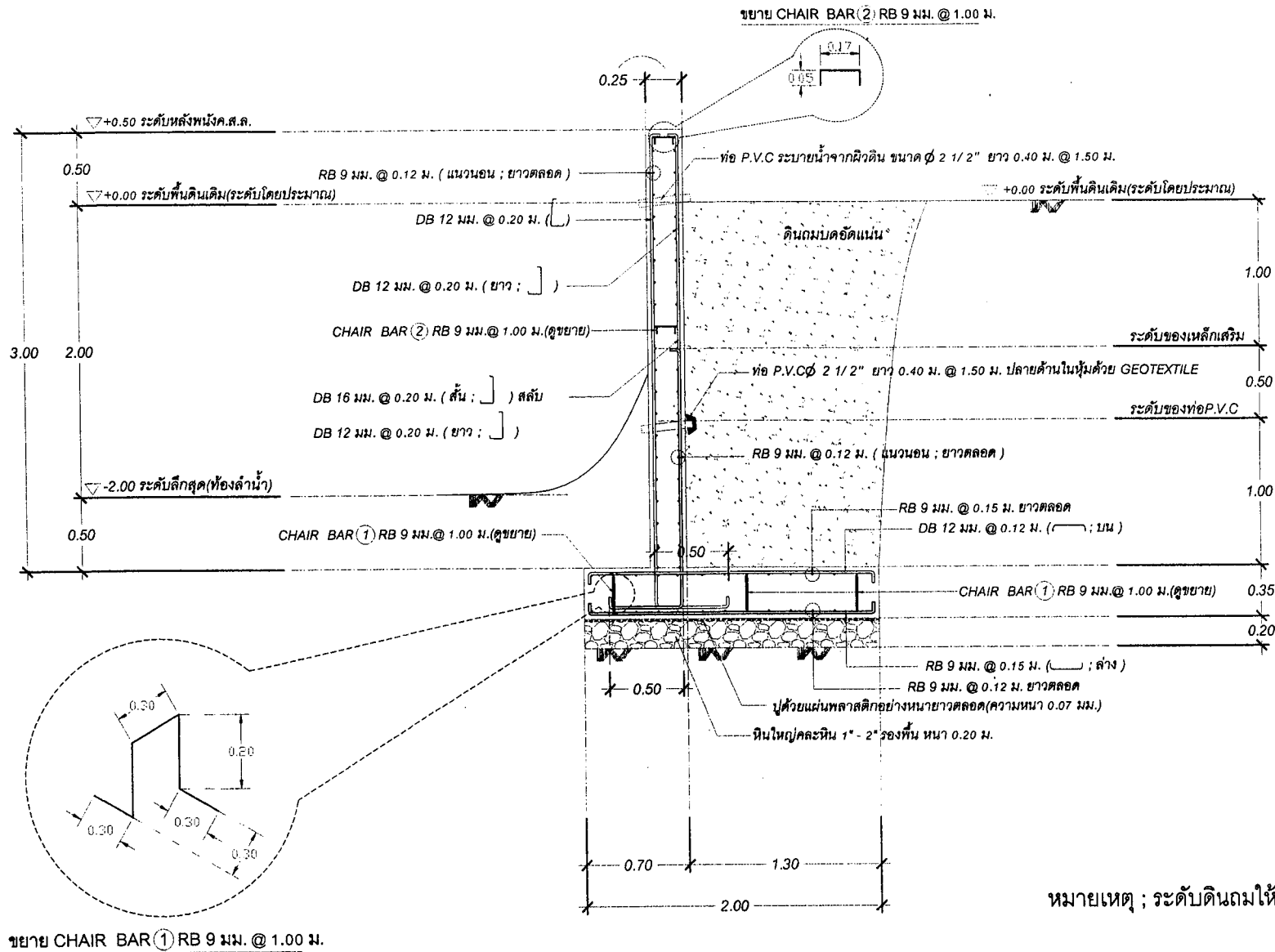
รูปตัด A-A ผนังกันดินคอนกรีตเสริมเหล็ก
